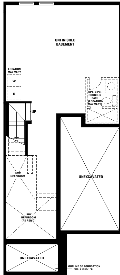
BASEMENT ELEV. 'A' & 'B'
