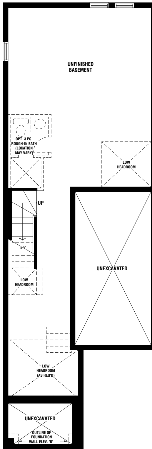
BASEMENT ELEV. 'A', 'B' END UNIT
