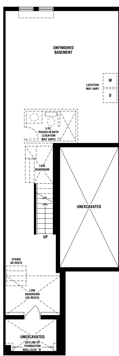
BASEMENT ELEV. 'A' & 'B'
